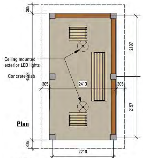
2 Smoking Shelter A2 Scale: 1:50
